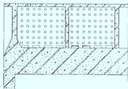
図5-38 有孔整流壁の例
